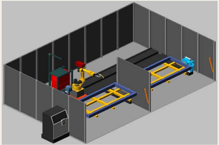
↑ Рис. 2. Схематичное изображение комплекса РК759.
